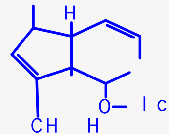
aucubi n
