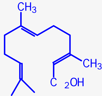
Farnesol
